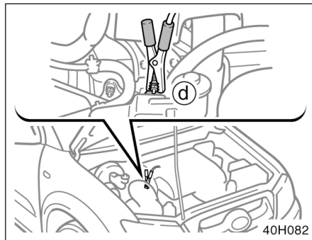
Ponto de conexão para motor 1KD-FTV
