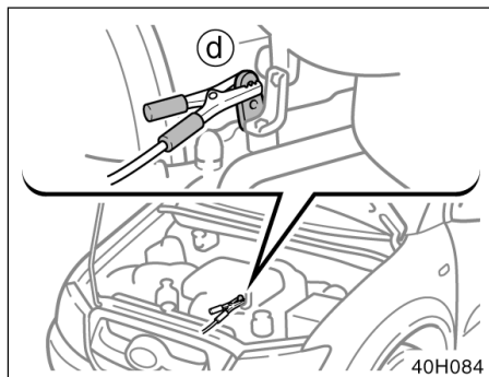
Ponto de conexão para motor 2KD-FTV
